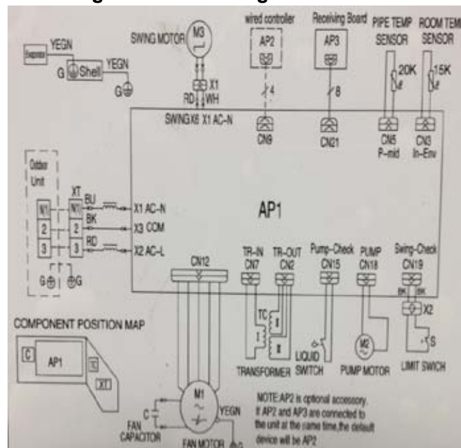
Diagramme de câblage du 24K :
